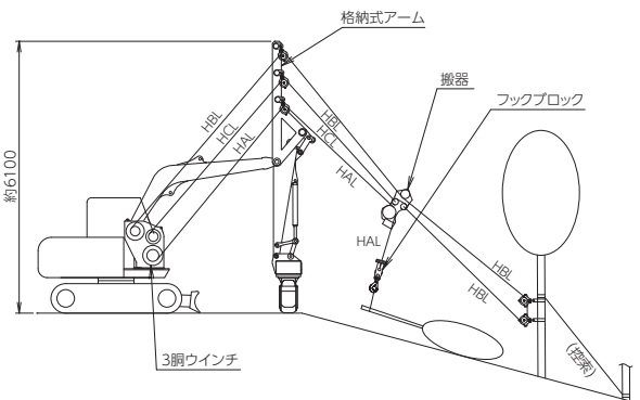
[設置・基本索張り図]
