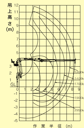
PL-960BL 作動線図
