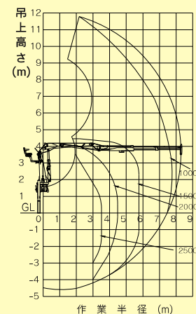
PL-860A 作動線図
