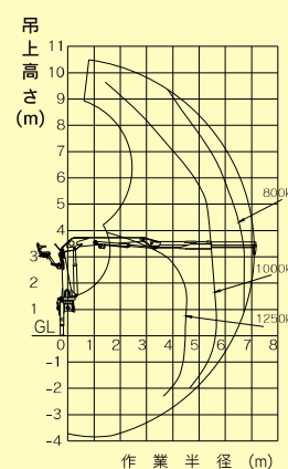
PL-660 作動線図
