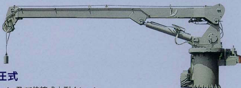
1.5t×6m 1本ブームクレーン
